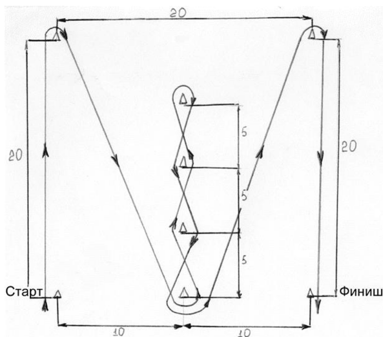
Рисунок 3 - Схема дистанции контрольного упражнения «Слалом»
